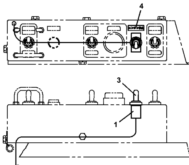
転倒警報付きの場合 WITH OVERTURNING ALARM
